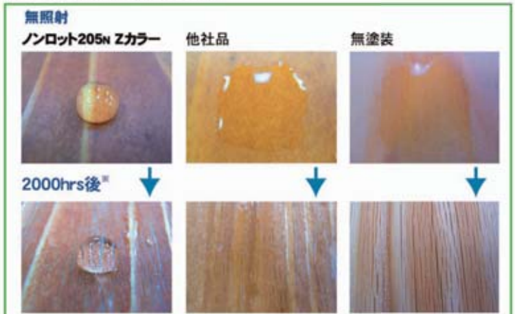
促進テスト結果 (杉板2回塗り)
